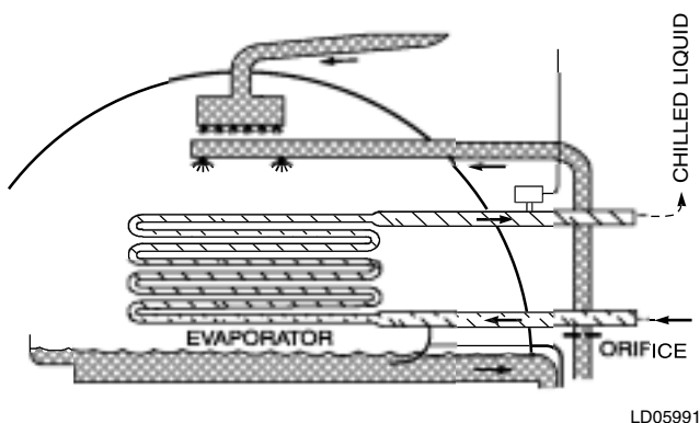
FIG. 5 – EVAPORATOR
