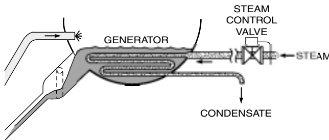
FIG. 8 – GENERATOR
