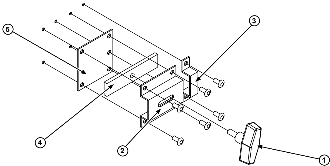
FIG. 4 - DOOR LATCH
