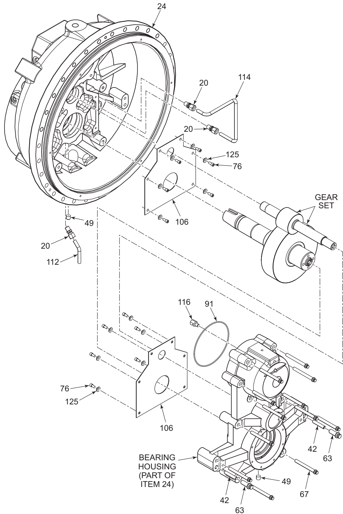
FIG. 11 - HF 41 COMPRESSOR
