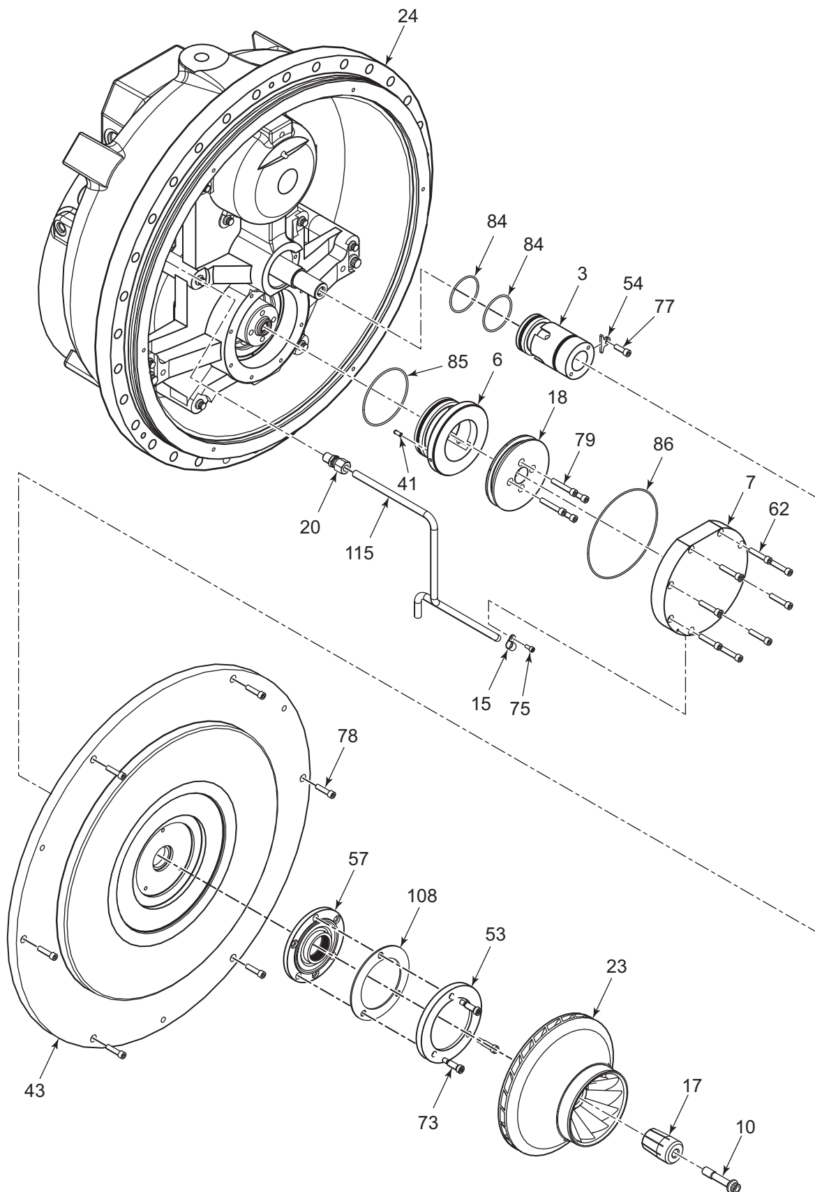
FIG. 10 - HF 41 COMPRESSOR
