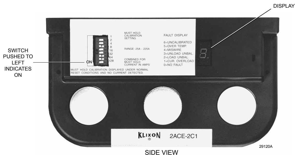
FIG. 45 – MOTOR PROTECTION MODULE
