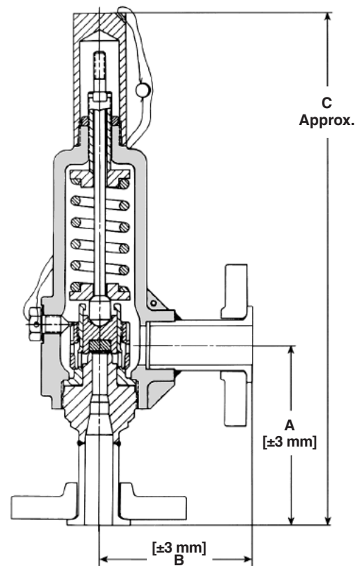
Flange x Flange
