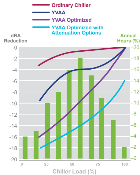
YVAA Sound Values vs. Ordinary Chiller
