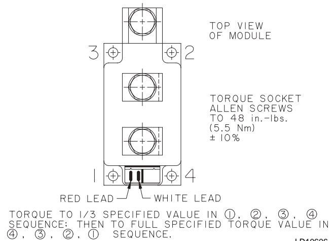
FIG. 14 – ISCR / DIODE MODULE TORQUE SEQUENCE
