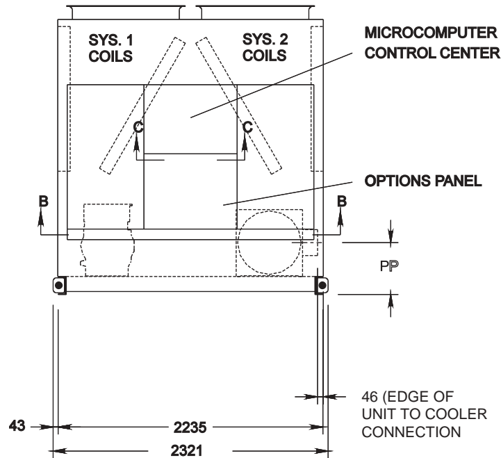
VIEW A-A
