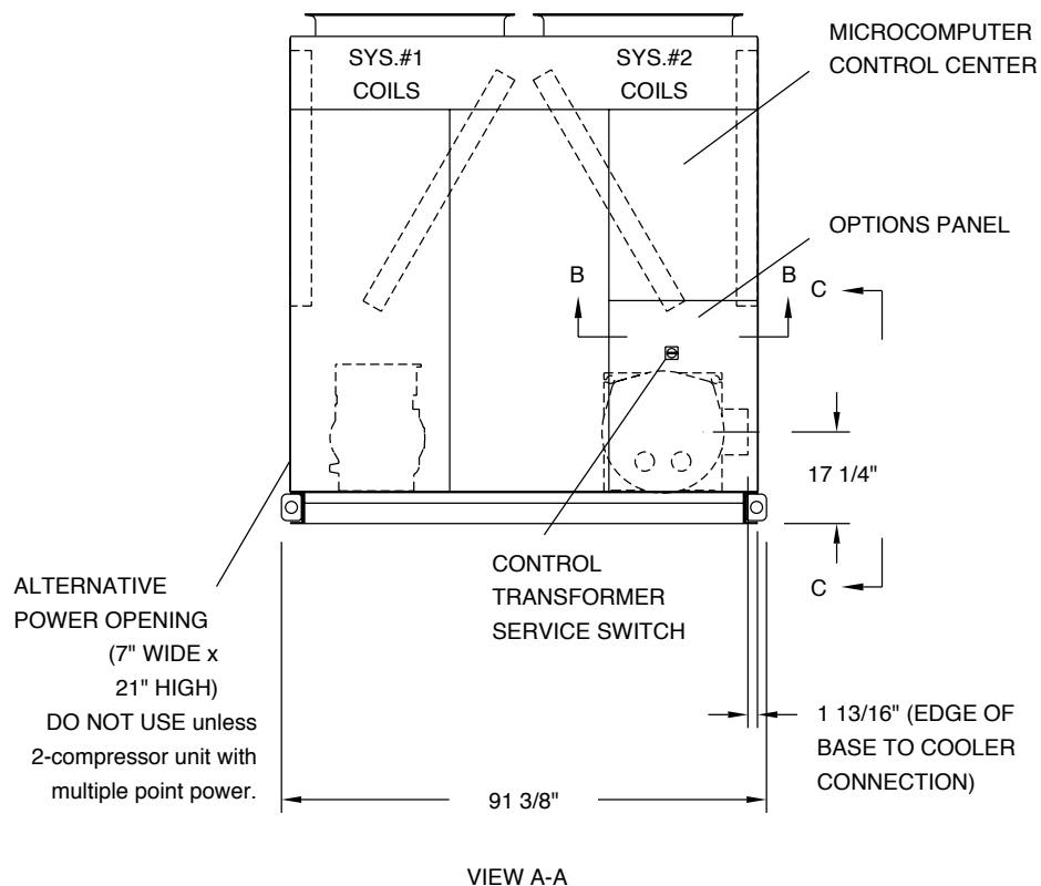
VIEW A-A
