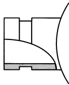
FIG. 6 – VICTAULIC GROOVE
