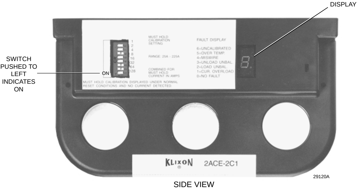
FIG. 36– MOTOR PROTECTION MODULE
