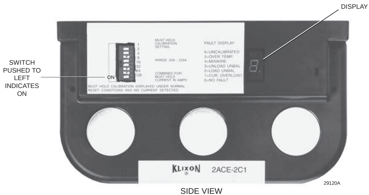
FIG. 40 – MOTOR PROTECTION MODULE
