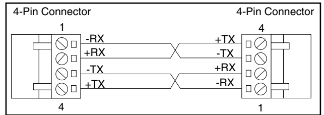
RS-422 Test Harness
