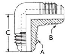
Union - Flare to Flare
