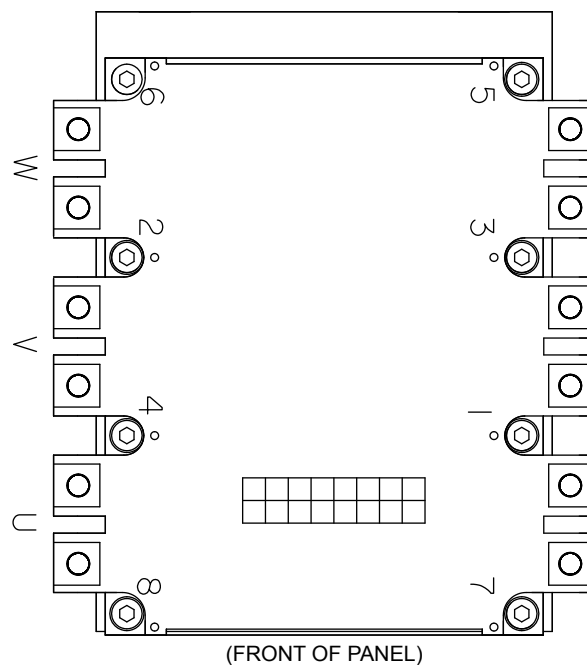
FIG. 20 - OSCD POWER MODULE
