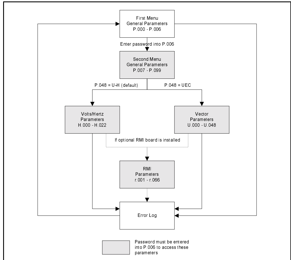
Figure 4.1 – Parameter Menu Structure
