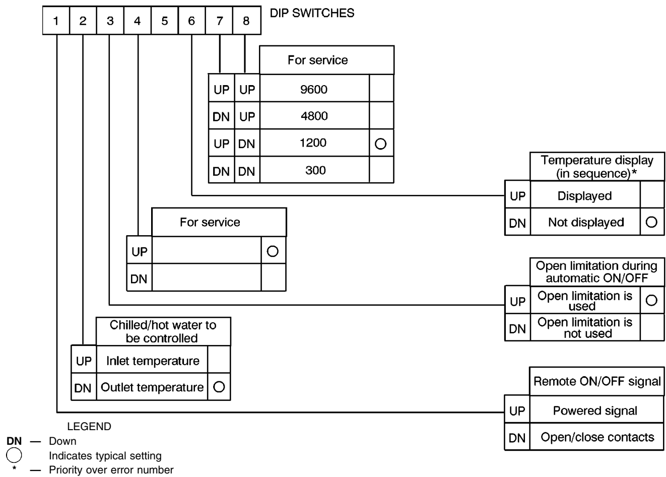
Fig. 16 — Switch SW11
