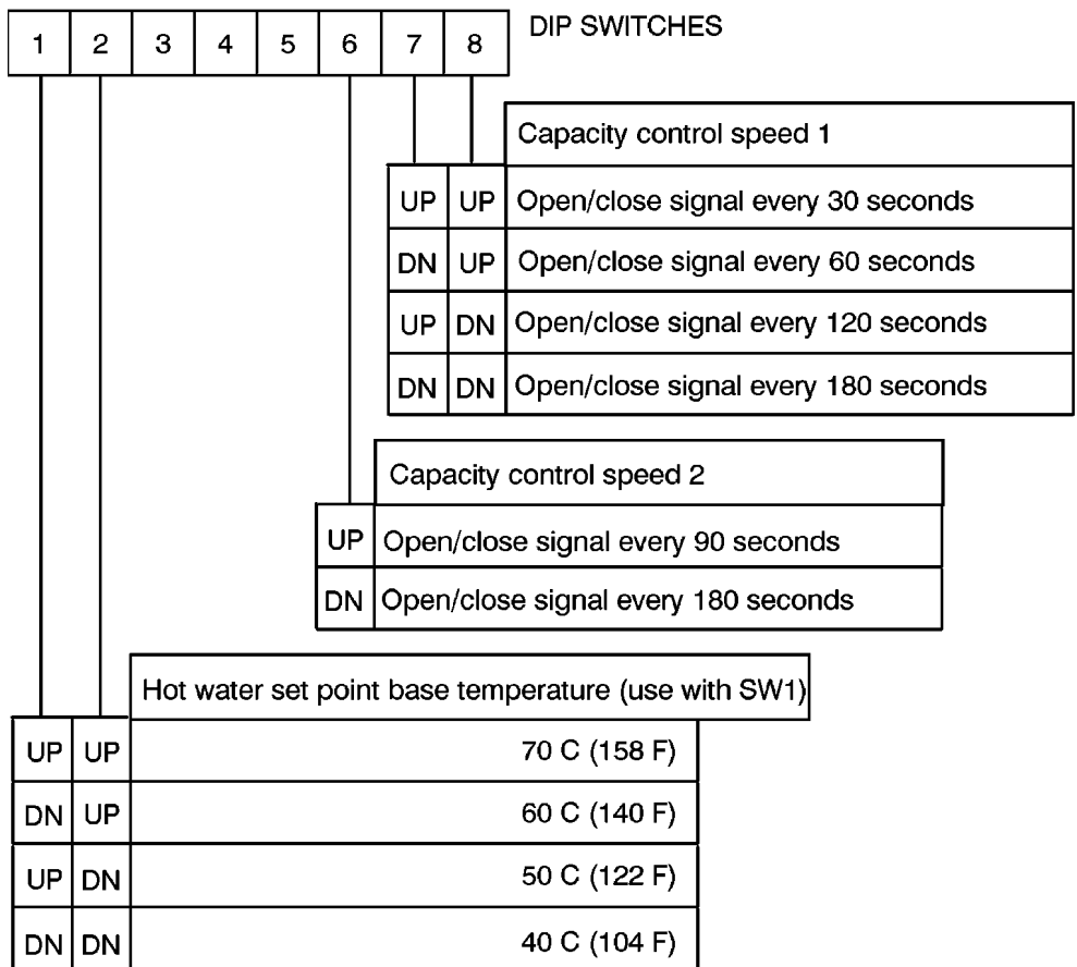
Fig. 15 — Switch SW10
