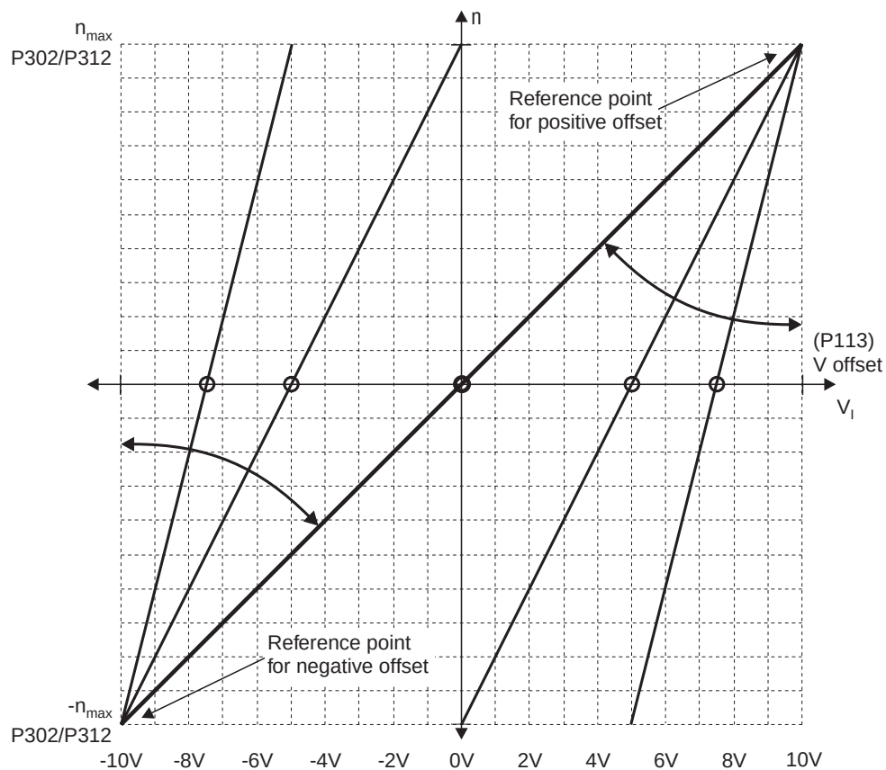
Fig. 53: AI1 voltage offset
