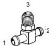
BFL-806 - Tee (1) (2) Hose Barb (3) Male Inv. Flare Swivel
