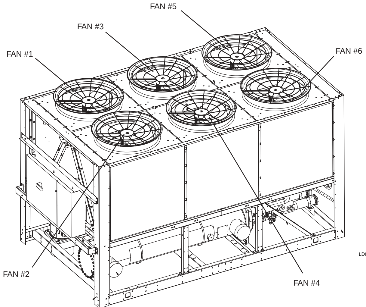
FIG. 10 – DYCAL0045 FAN LOCATION
