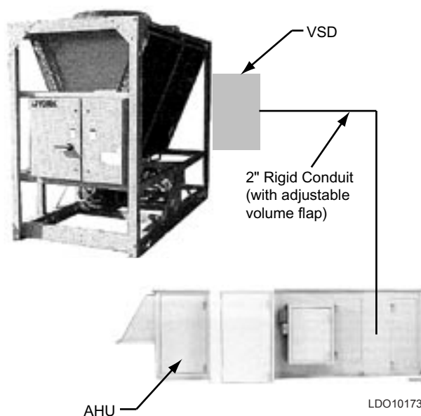
FIG. 14 – VSD VENTILATION
