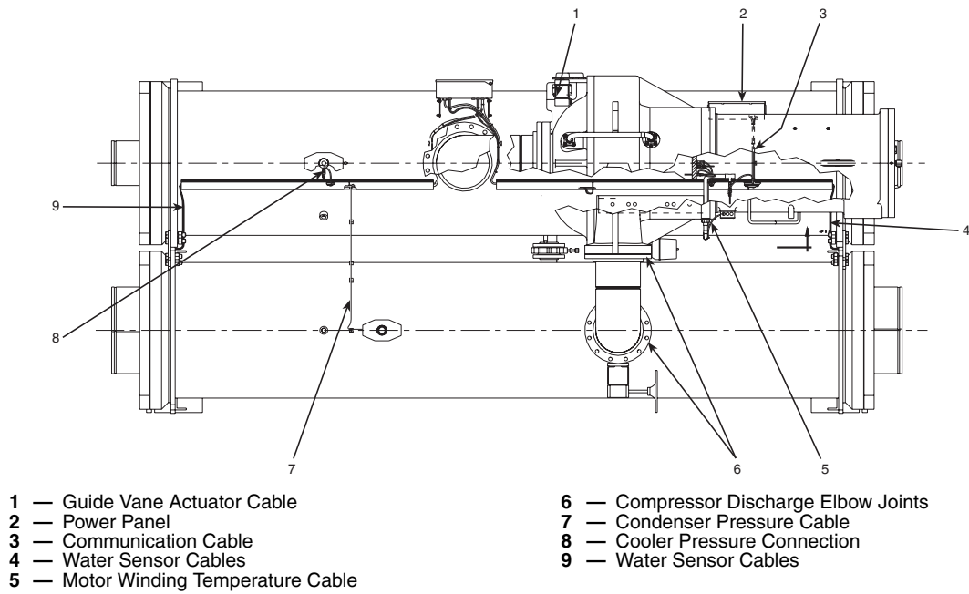
Fig. 9 — 19XR Chiller Top View
