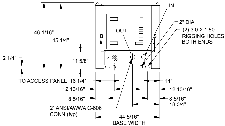
LEFT END
